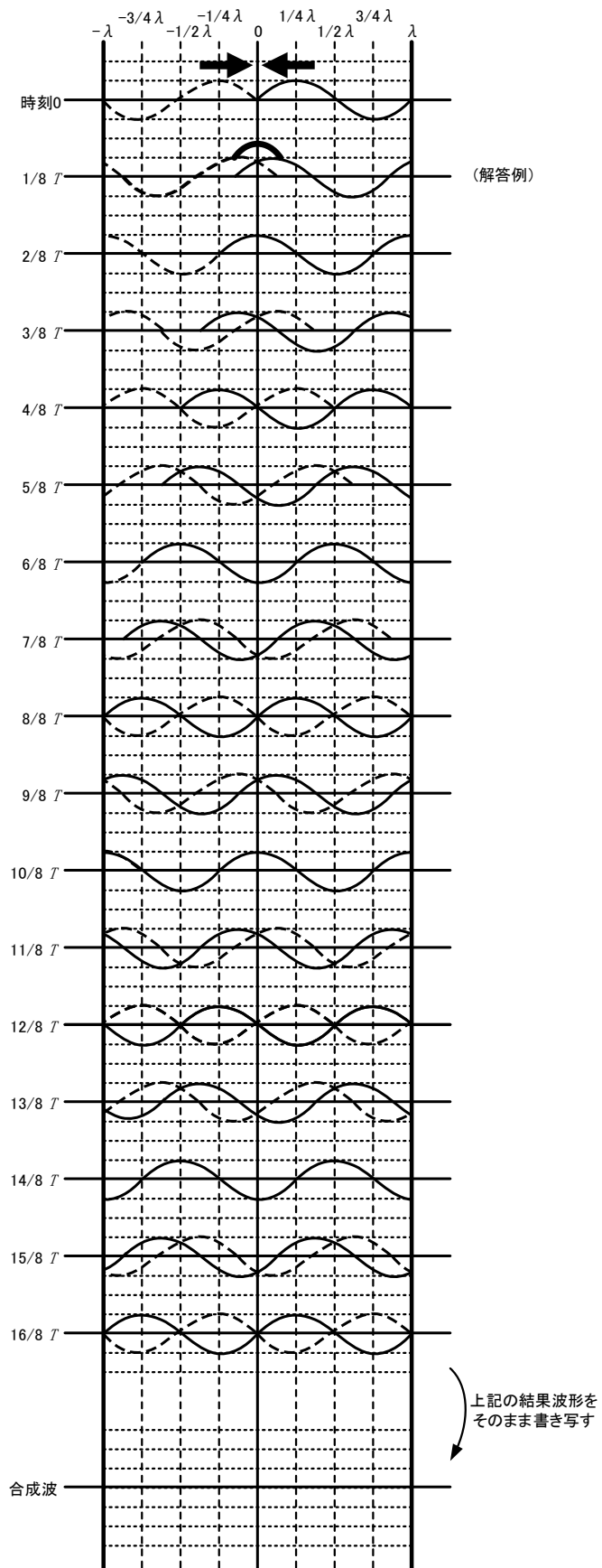
図 2つの波が重なった波と合成波 (1/8周期 = \pi/4\omega ごとの波形)
